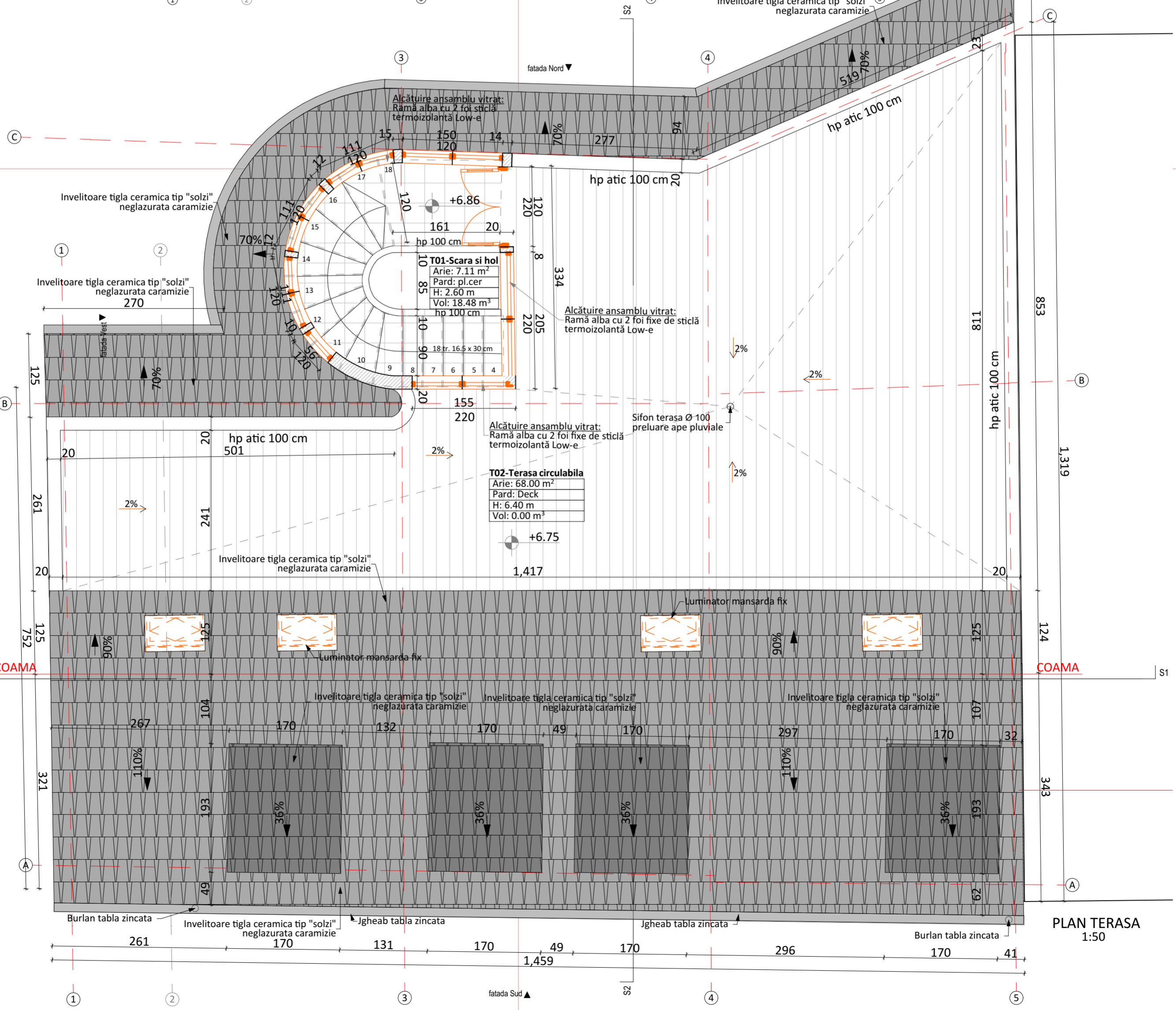
PLAN INVELITOARE 1:100
